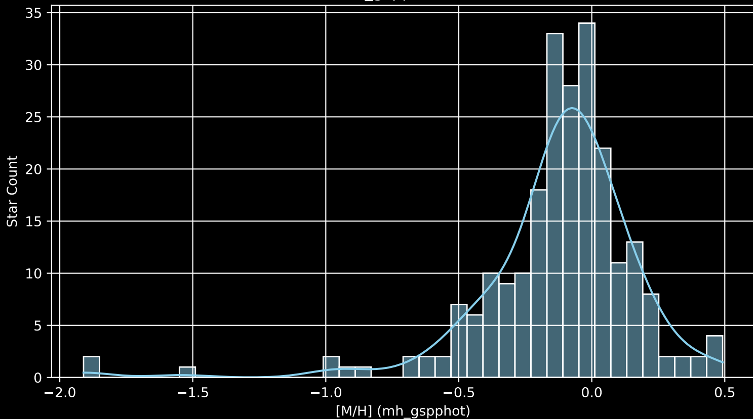
APOGEE DR17 Field: [281+12 [M/H] (mh_gspphot) (n= 232)
