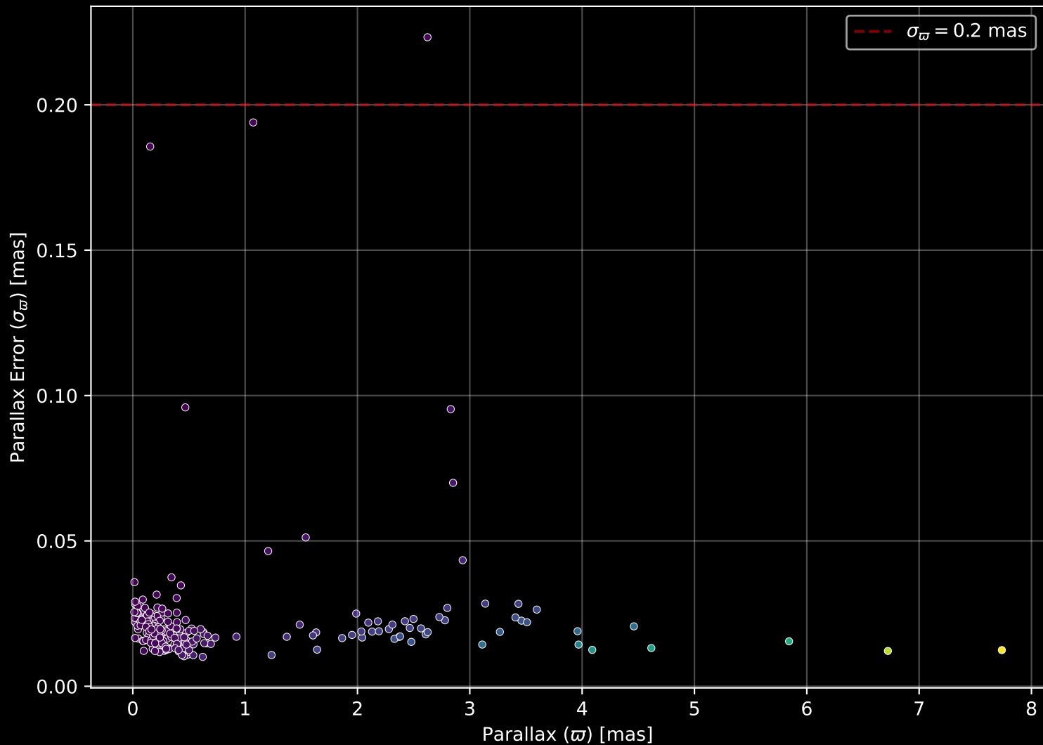
APOGEE DR17 Field: [281+12] Parallax Quality (n= 237)
