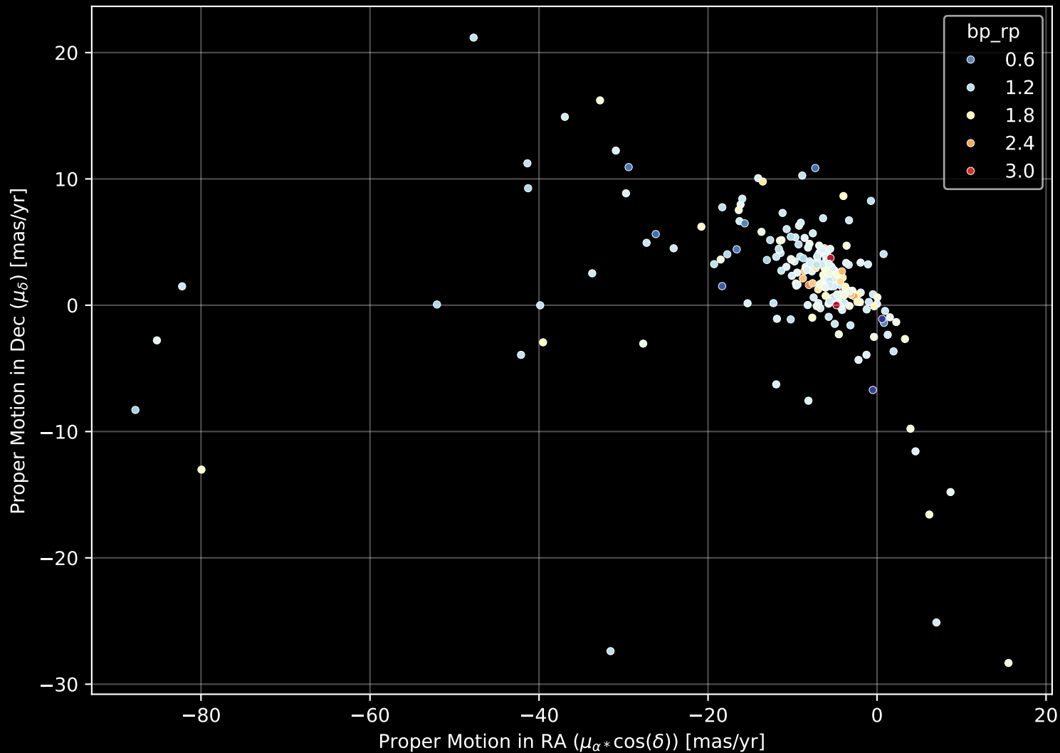
APOGEE DR17 Field: [281+12] Proper Motion Diagram (n= 237)
