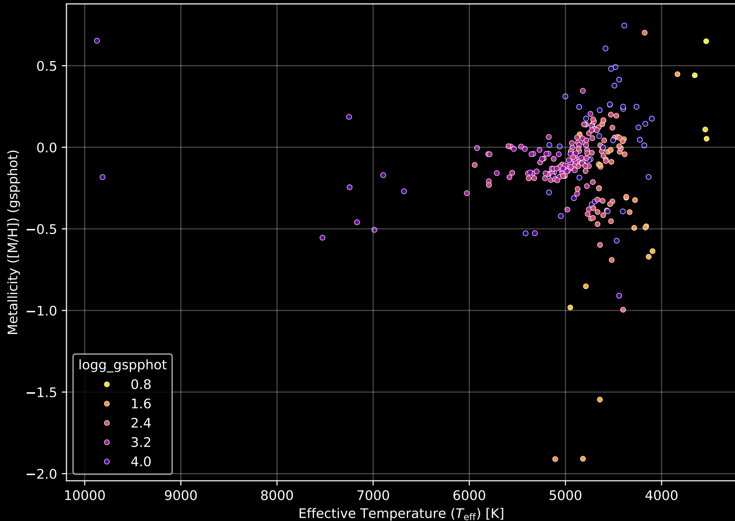
APOGEE DR17 Field: [281+12] Stellar Population Parameters (n= 237)
